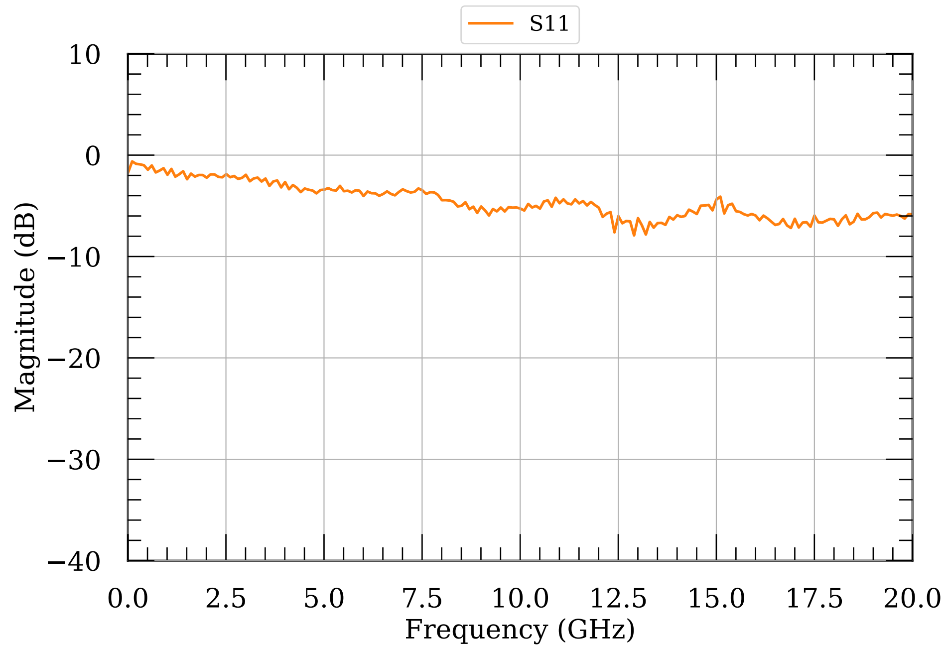
LNA S-params module013
